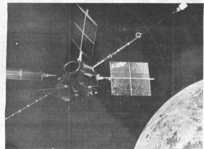
Este imaginario dibujo muestra al laboratorio científico Explorer 35 tal como se supone que se colocará en órbita lunar. La astronave fue lanzada el 19 de julio desde Cabo Kennedy, Florida. Pesa 100 kilogramos y está diseñada para recoger y transmitir a la Tierra datos sobre la radiación, los vientos solares, el polvo espacial, las fuerzas magnéticas y otros fenómenos especiales que ocurren en la proximidad de la Luna. Se espera que esta información tenga gran valor para proyectar los futuros vuelos tripulados a la Luna.
