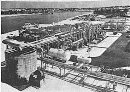
Vista general de una planta de desalación que se acaba de construir en Cayo Hueso, Florida. La planta que costó 3.399.000, dólares, la manejarán cinco trabajadores. Convierte unos 6 millones de galones de agua marina en 3 millones de galones de agua potable.
