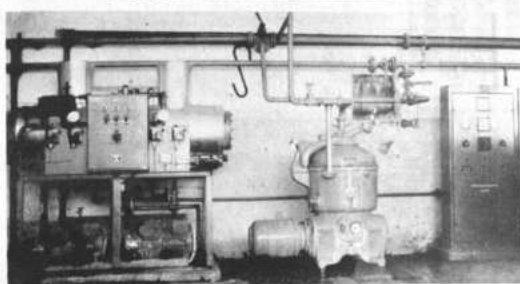
Varios aspectos de la nueva máquina de mercerizar que, a un costo de 100.000 dólares ha sido instalada por SAID S. A.
