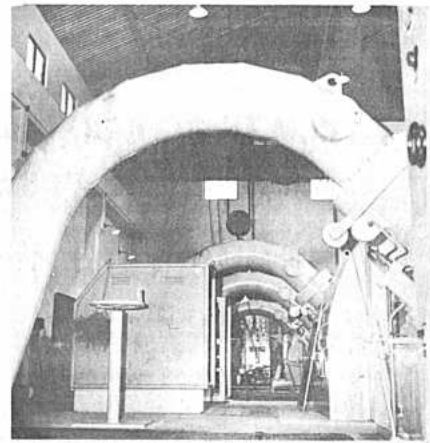
Vista de las dos máquinas hidroeléctricas de la nueva plantación Chururiqui que desarrolla una potencia de 26.000 kilovatios. En la ciudad de La Paz, se está desarrollando un programa de gran amplitud en el sistema eléctrico de distribución, así como en las diferentes sub-estaciones se ha aumentado la potencia para una adecuada distribución de la energía disponible.
