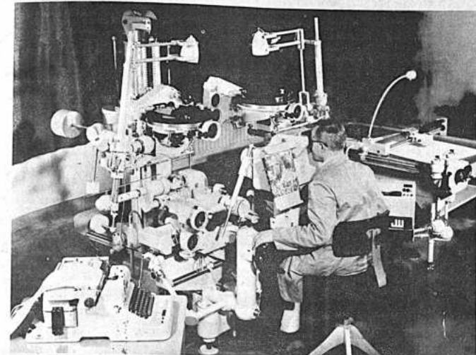
DE LA PELICULA AL PLANO DE PLANCHETA.- Un problema para cuya resolución científicos y de- licuentes necesitan varias semanas lo realiza hoy una máquina en varias horas. El aparato cartografi- co, reproducido en nuestra foto, transmite fotografías aéreas a planos de planchetas. Este estereopla- grafo que está conectado con una instalación registradora de coordenadas, electromagnética, y el cual fue exhibido en la última feria de Hannover por la firma Carl Zeiss en Oberkochen (Rep. Fed. de Ale- mania) cumple todas las condiciones para una cartografía exactísima, a escala, a base de aerofotos.
