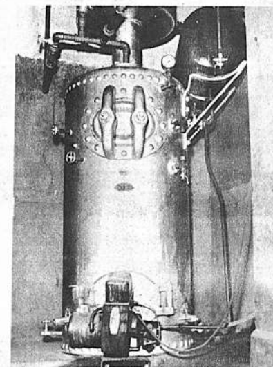
Caldero de alta presión para suministro de vapor a las máquinas.
