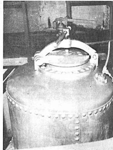
Auto-clave para producción de harina de hueso.
