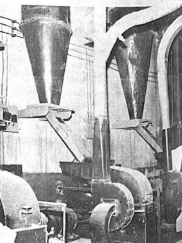
Equipo de molino para producción de alimentos balanceados.
