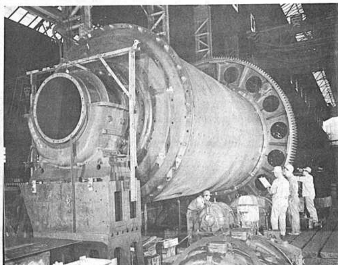
Molino de cemento (en fabricación)
