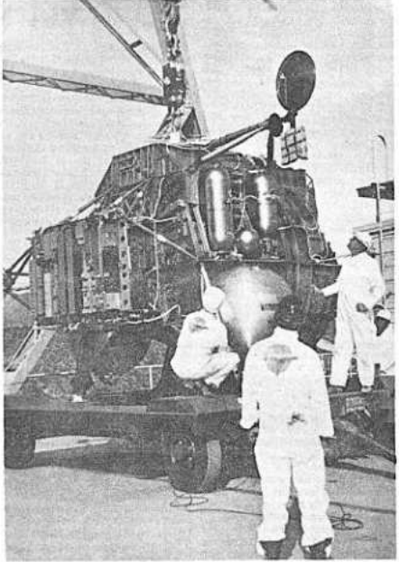
PLATAFORMA DE PRUEBA DE LA NAVE "LUNAR MODULE". La sección de ascenso de la nave espacial para el vuelo lunar tripulado es objeto de pruebas en una plataforma al aire libre en White Sands, Nuevo México. El vehículo se está perfeccionando y ensayando para emplearse en el Programa Apolo de descenso en la luna. Dos de los tres astronautas abandonarán la nave principal de comando, que se mantendrá en órbita de luna, y descenderán a la superficie de la luna. Los cohetes en el momento de descenso, se dispararán para hacer regresar a los dos astronautas a la astronave de comando para el vuelo de regreso a la tierra.
