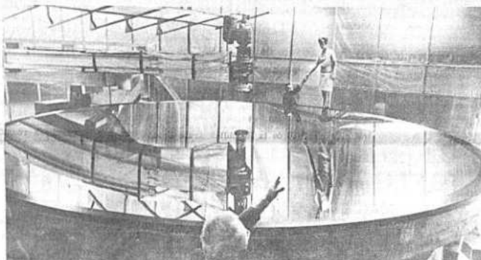
ESPEJO DE CAMARA ESPACIAL. Este inmenso espejo será utilizado en el Jet Propulsion Laboratory, de California, para duplicar la intensidad del sol fuera de la atmósfera de la tierra, en las pruebas de naves espaciales. El reflector de siete metros de diámetro proyectará luz artificial a intensidad solar sobre una cámara de vacío super-belada, para aproximarse a las condiciones del espacio exterior. El espejo, de aluminio con una capa de níquel es casi dos metros más grande que el usado en el telescopio reflector más grande del mundo, en lo alto del Monte Palomar, en California.
