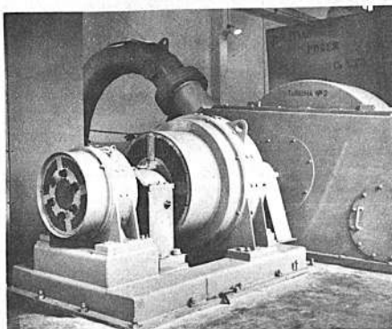
La máquina de Excitación de la Unidad No. 2.
