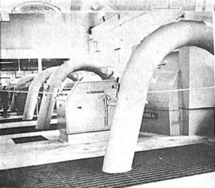
Vista de las 2 Unidades de la Planta Hidroeléctrica de Chururacui, que desarrolla una potencia de 23,000 KWS.
