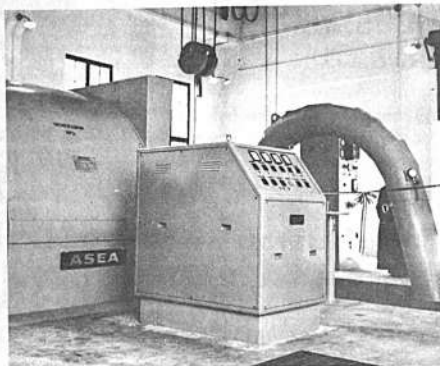
Gobernador automático que controla la Unidad No. 2 de Chururacui.
