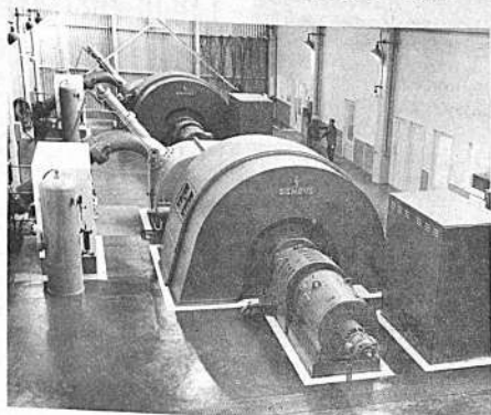
Dos inmensos generadores en pleno funcionamiento en la casa de máquinas en Pampa Tambo.
