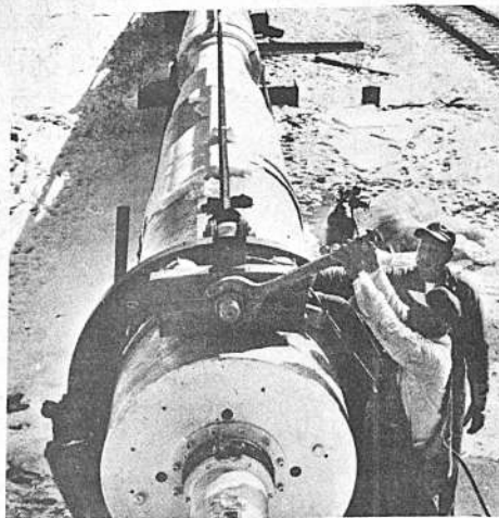
CAÑÓN DE INVESTIGACION. Este artefacto de la Marina de Guerra de los Estados Unidos, que se construye en Virginia, tiene por objeto estimular los efectos de las ondas producidas por las explosiones nucleares, sin el uso de materiales radioactivos. Consiste en cuatro cañones de barcos de guerra, unidos, y un tubo de casi un kilómetro de largo. Se hace explotar un explosivo dentro del primer cañón, y la fuerza resultante es amplificada 40.000 veces, mientras se dirige a una velocidad de diez veces la del sonido hacia el extremo del tubo. Dentro de este hay equipos de investigación y las cámaras registran los movimientos mientras que nadan las ondas. La mayor parte de la fuerza es absorbida antes de llegar al extremo del tubo.
