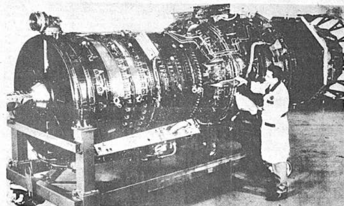
MOTOR DE TRANSPORTE SUPERSONICO. Este es un prototipo del motor turbojet GB4 que construyó la compañía General Electric, de Schenectady, en los Estados Unidos, para el avión de transporte supersónico norteamericano. Cuatro de estos motores servirán para impulsar a este avión de 350 pasajeros, que se espera esté en servicio comercial para 1974. Este tipo de motor, tiene una longitud de 7,5 metros y desarrollará una energía propulsora de 27.000 kilogramos, tres veces más que la de cualquier avión comercial de propulsión a chorro.
