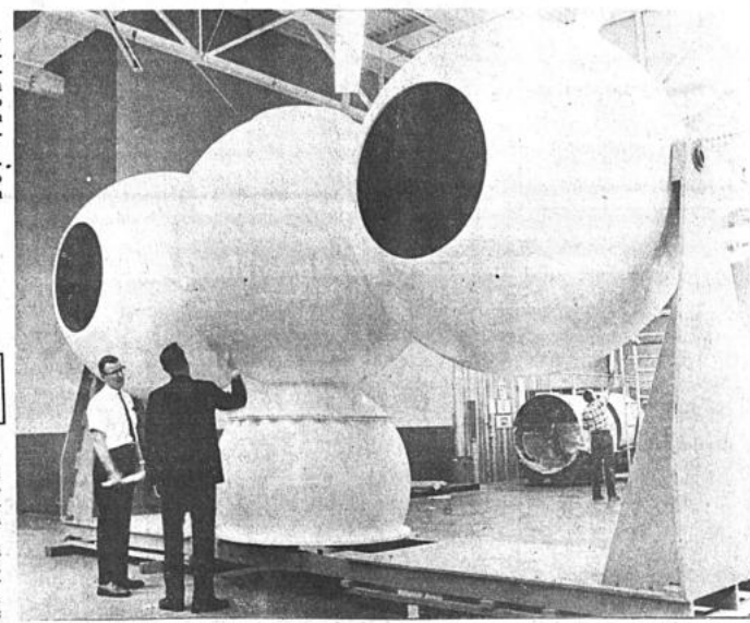
California.- Estas son las tres esferas de intercomunicación que serán introducidas en un proyecto submarino. Tienen una capacidad de presión máxima, calculada en 3.500 pies de inmersión. Estarán equipadas con botones de contacto y adyacentes de transferencia de energía.
