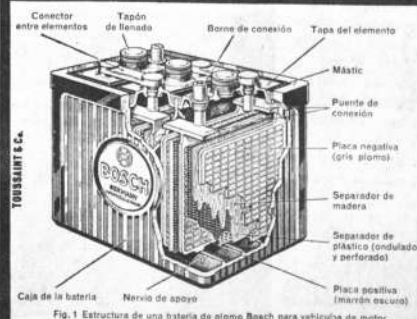
Fig. 1 Estructura de una batería de plomo Bosch para vehículos de motor
