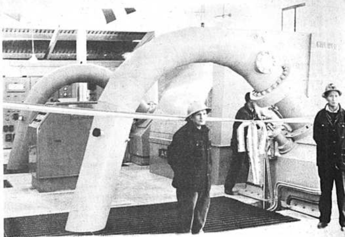
Sala de máquinas de la planta de Chururaqui, en Zongo, donde funciona la primera unidad de 11.500 Kws. En la misma sala, la mitad del espacio está destinada a la instalación de la segunda unidad de 11.500 Kws. que, según se afirma ahora, será inaugurada en octubre. Las máquinas de manufactura europea, son las más modernas en su tipo y operan mediante controles eléctricos y automáticos.
