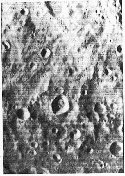
Esta es la primera fotografía que Estados Unidos obtuvo del lado oculto de la Luna, mediante la cámara de alta resolución que lleva el Orbiter Lunar. La foto fue tomada el 21 de agosto y transmitida a la estación de Goldstone. La foto cubre un área de 75 a 100 millas de superficie lunar. (AP Wirephoto)
