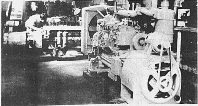
Maquinaria pesada para movimientos de tierra, grupos electrógenos y maquinaria agrícola constituyen la principal importación de CIBO. Cafeteros y arroceros de Santa Cruz de la Sierra han adquirido más de 55 tractores.
