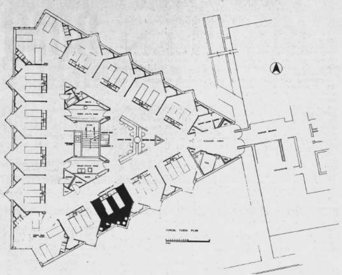
El plano del Pabellón Lane del Hospital de Point Pleasant de New Jersey muestra cómo se presta la forma triangular a la eficiencia en el funcionamiento y a la reducción de las áreas destinadas a los servicios centrales. Además, las líneas rectas del edificio reducen los gastos de construcción en relación con las formas circulares.
