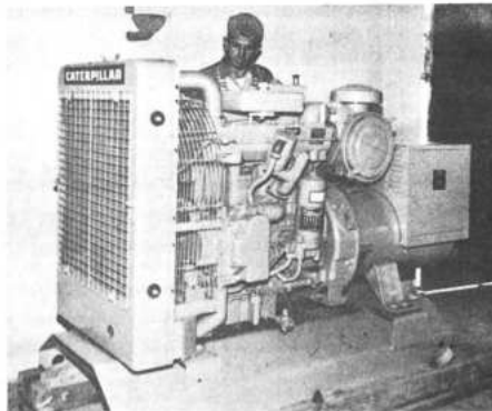
Este es el motor de luz de Montequidá provisto por la Alcaldía Municipal. Otro igual fue proporcionado a la población de Tarabuco.
