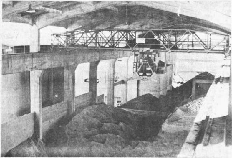
HANGAR DE CALIZA, ARCILLA, CLINKER Y YESO.
