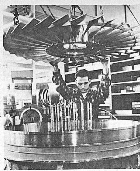
EL TITANIO USADO EN UN MOTOR DE PROPULSION A CHORRO. La pieza de este motor está hecha de titanio, el nuevo metal de la era del espacio, y va a ser instalada en el compresor de un motor a chorro Pratt y Whitney JT4. Las paletas producen un 30 por ciento más de fuerza motriz en los motores a chorro que la desarrollada por los de diseño corriente.
