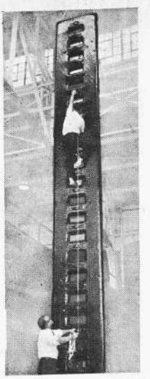
ESCALERA DE LA ERA ESPACIAL.- Ingenieros de la Goodyear prueban una escalera inflable, la cual será usada dentro de los tanques de combustible del cohete lunar Saturn V. Esta escalera se enrolla en un pequeño paquete para sumergirla a través de la abertura del tanque, la cual es suficientemente grande como para que entre un hombre, pero muy pequeña para introducir una escalera normal. Este diseño de goma mide alrededor de 8 metros de largo y es inflado dentro de los tanques.
