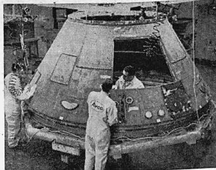
BLINDAJE TERMICO PARA EL APOLO. Tres expertos de la planta de Avco, de Lowell, Massachusetts, terminan de armar el blindaje térmico para la astronave Apolo. El blindaje se compone de 350.000 celulas a manera de panel llenas de un material aislador y protegidas a los tres astronautas de la tripulación del efecto de las temperaturas sumamente altas generadas por la fricción atmosférica durante el trayecto de regreso de la nave a la tierra después de su vuelo de exploración lunar.
