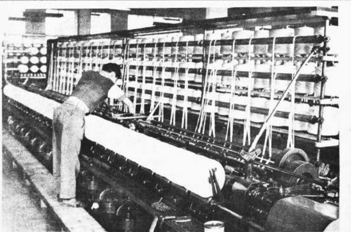
LA HILANDERIA de lana peinada, donde la materia prima recibe un trato muy cuidadoso para lograr la fibra más fina que es utilizada en la fabricación de casimires y paños. Al respecto, dentro de tres meses, la fábrica iniciará la confección de mercadería de nuevo acabado, resistente a la humedad inarrugables, que compita sin desventaja alguna con los productos que son importados actualmente.
