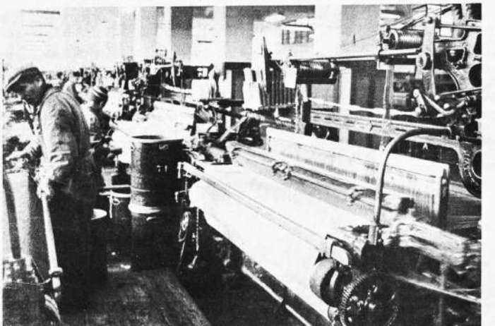
LAS FIBRAS sintéticas de procedencia alemana son mezcladas con lana nacional para la fabricación de paños, mantas y otras telas, obteniéndose productos resistentes. La fábrica, actualmente, cumple un horario de trabajo que se inicia a las 7 de la mañana y concluye a las 16 horas. Hay la confianza de que en el futuro puedan aumentarse los turnos, de acuerdo a las demandas del público.
