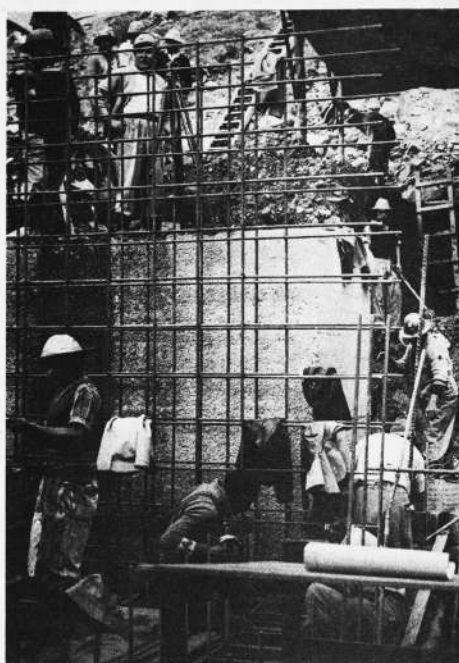
Sólidas estructuras de concreto armado se preparan en "Pampa Tambo" para la instalación de las turbinas que generarán 27.000 kilovatios al cumplirse la primera fase del proyecto hidroeléctrico de Corani, financiado por el BID, el Banco Mundial, dentro de la Alianza para el Progreso.
