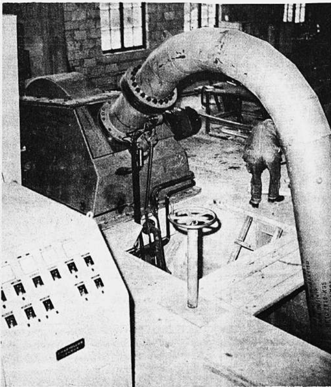
La presente fotografía muestra la tubería de entrada a la turbina, junto al tablero de control del gobernador, se puede apreciar el tipo de diseño completamente moderno.
