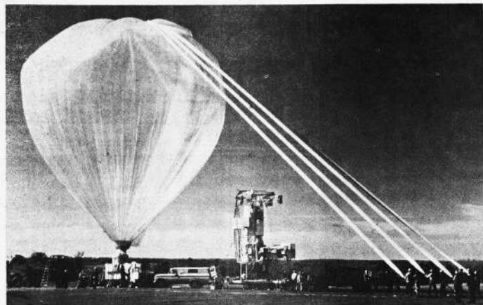
PREPARATIVOS PARA EL LANZAMIENTO -- Cuatro tubos de helio comprimido llenan el globo auxiliar del Estratoscopio II norteamericano poco antes de que éste suelte amarras en la estación de globos para vuelos científicos establecida por el Gobierno de los Estados Unidos en la población tejana de Palestine. El enorme telescopio que irá suspendido del globo aparece en el centro de la fotografía sobre la plataforma de un cañón. Las vistas tomadas desde las altas capas atmosféricas muestran más detalles de los cuerpos celestes que las captadas hasta ahora con telescopios desde la Tierra (No. 65-1667.)
