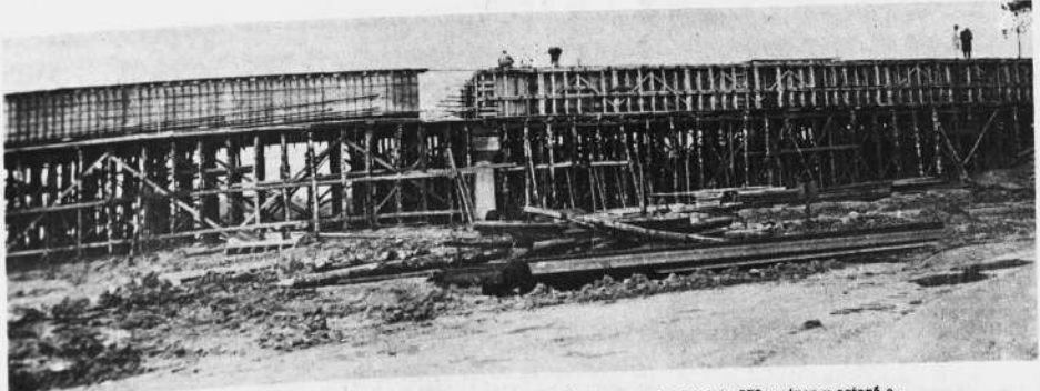
Parte del puente que se construye sobre el río Yapaní. Tiene una longitud de 572 metros y estará asentado en su conclusión sobre 14 pilares de 7 1/2 metros de ancho los mismos que se encuentran asentados a una distancia de 39 metros. El costo aproximado para la conclusión total de este puente está calculado en dos millones de dólares. Los técnicos estiman que la obra será entregada entre mayo o junio del próximo año.
