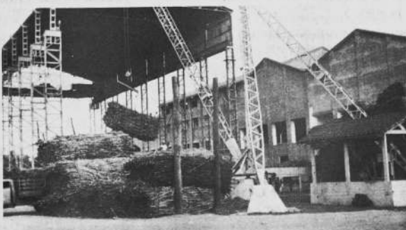
El estibaje de la caña en el barracón del Ingenio San Aurelio, que tiene una capacidad para seis mil toneladas. El barracón es otra de las modernas instalaciones con las que se ha logrado acelerar la producción azucarera.
