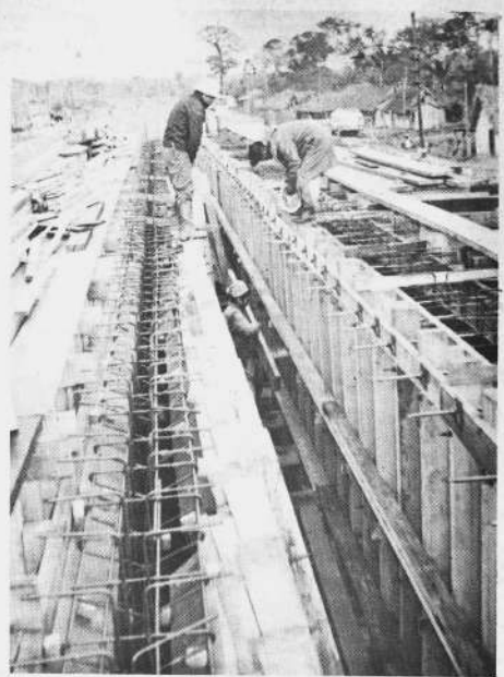
Esta es una parte de las vigas que forman el armazón del puente sobre el río Yapacaní. Es una estructura que se levanta de acuerdo con los últimos adelantos técnicos.
