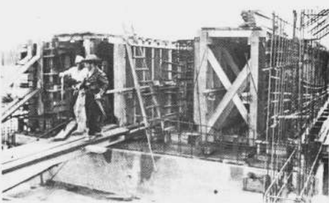
Puede observarse el encofrado del armazón del puente que tendrá una longitud de 572 metros, siendo el primer puente de este tipo que se construye en el país.
