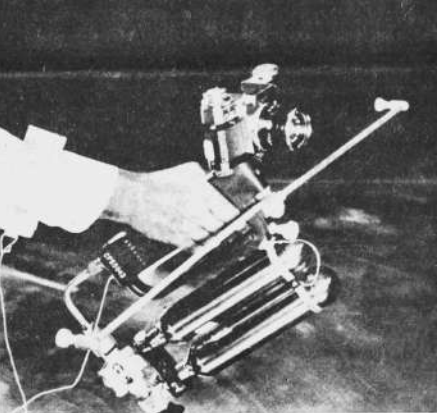
Esta es la pistola de propulsión a chorro que White utilizó para moverse libremente en el espacio durante los veinte minutos que estuvo fuera de la capsula. La pistola lleva una cámara fotográfica de gran precisión con la cual White tomó muchas fotos aún no dadas a publicidad.
