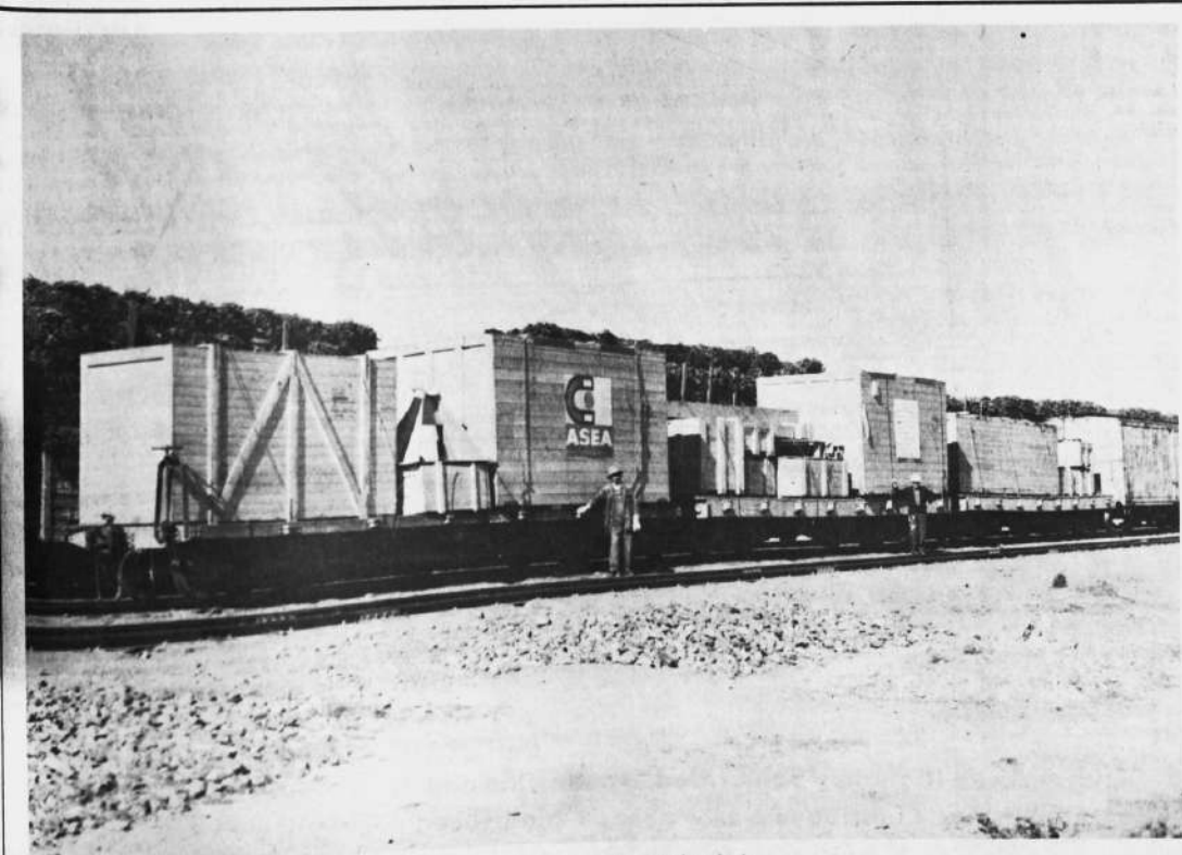
Este generador, con 14.500 kva. ha sido fabricado en Suecia por la Compañía "Asea", siendo el de mayor potencia existente en Bolivia hasta la fecha.
