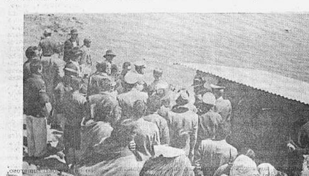
A la izquierda, la comitiva oficial y campesinos observan la represa de Melga con capacidad para regar 300 Hs. de tierra para cultivos. A la derecha, la represa de Totorá Kiocha, en Punata, con capacidad de riego de 600 hectáreas. Ambas obras han sido financiadas por USAID, los campesinos y el Plan de Desarrollo Rural.
