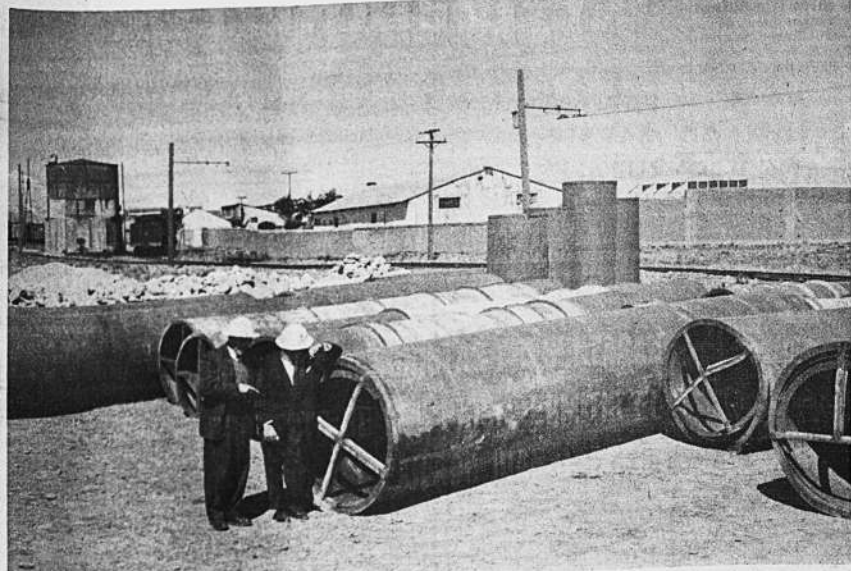
BOLIVIAN POWER COMPANY LIMITED, intensifica los trabajos de construcción en la nueva planta hidroeléctrica de Chururqui en el Valle de Zongo, que entrará en servicio en la primera etapa, aumentando 13.000 K.2. el sistema eléctrico actual de la ciudad, a fines del año en curso. La presente fotografía muestra la tubería de 1.40 mts. de diámetro fabricada en Brescia, Italia, que conducirá el agua a las turbinas de la indicada usina.
