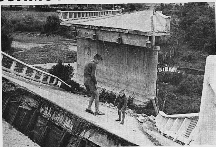
Enormes fueron los daños sufridos por varias regiones de Chile durante el terremoto que asoló a este país el 28 de marzo pasado. Esta fotografía da una idea de la violencia del sismo. Se trata del puente Pu-llalli, en la Carretera Panamericana Norte, frente al desvío a Zapallar, que tiene destruido un tramo completo, el cual cayó al estero del mismo nombre, a 10 metros de profundidad. La ruptura de este tramo obligó a los vehículos a realizar grandes rodeos para llegar a destino.
