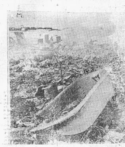
ESTE es el estado en que quedaron algunos tubos de conducción de gas, después de la explosión que se produjo en un área residencial en la población de Natchitoches, Louisiana, causando la muerte de 17 personas y la destrucción de cinco casas. (AP Wirephoto).
