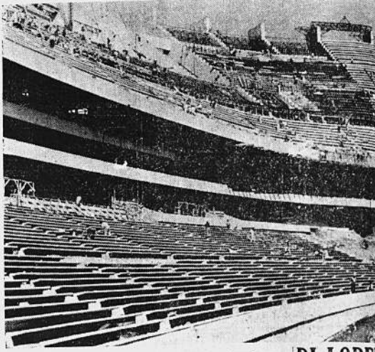
GRAN ESTADIO.— Este es el estadio, en plena construcción, que presentará México en los Juegos Olímpicos de 1968. Tendrá una capacidad para 110.000 espectadores. (AP Wirephoto).
