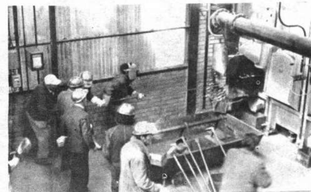
-Dos aspectos de la ceremonia de inauguración de la fundición de bismuto cumplida en el interior de la planta. Arriba, el encargado jefe de producción coloca al Gerente de COMIBOL los guantes y mandil de protección para la primera colada de metal. Abajo, procedimiento electrolítico para iniciar la sangría.
