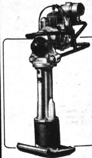
APISONADOR VIBRADOR WACKER BS-50
