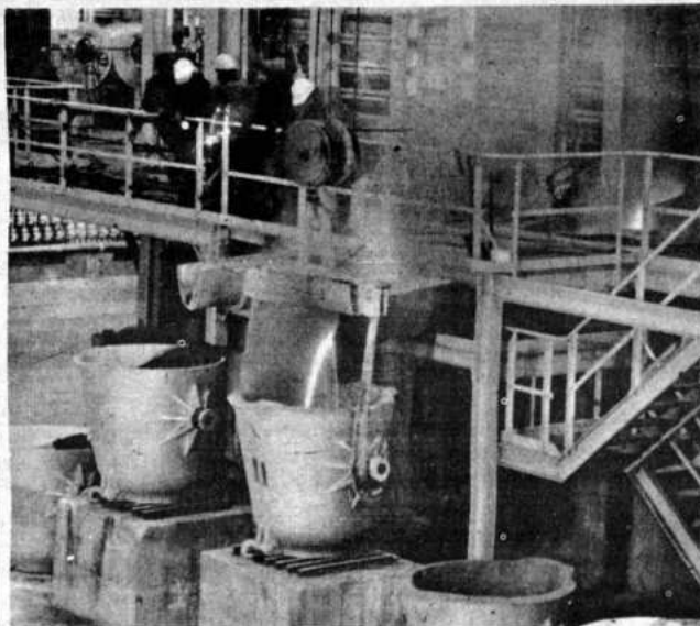
Un aspecto de la sangría en el horno de fusión del gigantesco complejo metalúrgico de Vinto, Oruro.
