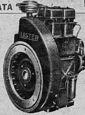
TIPO HR-2 29,5 HP - 2200 RPM
