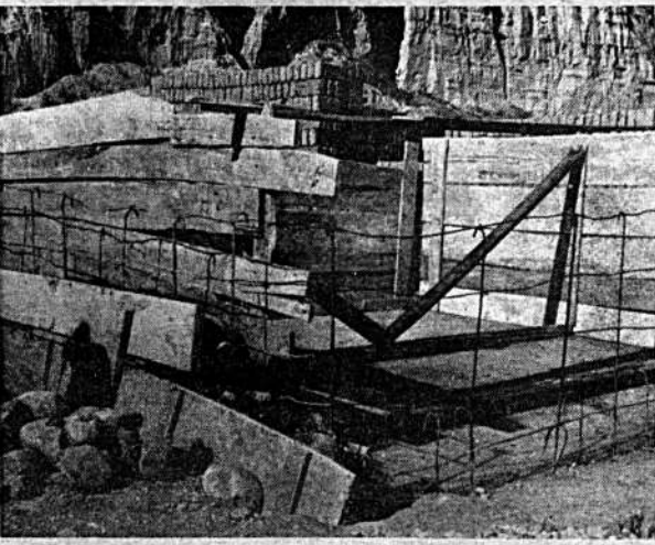
En Villa Jucumarini se construyen tanques para agua potable donde los vecinos contribuyen con su propio esfuerzo y el asesoramiento de técnico de Acción Comunal.
