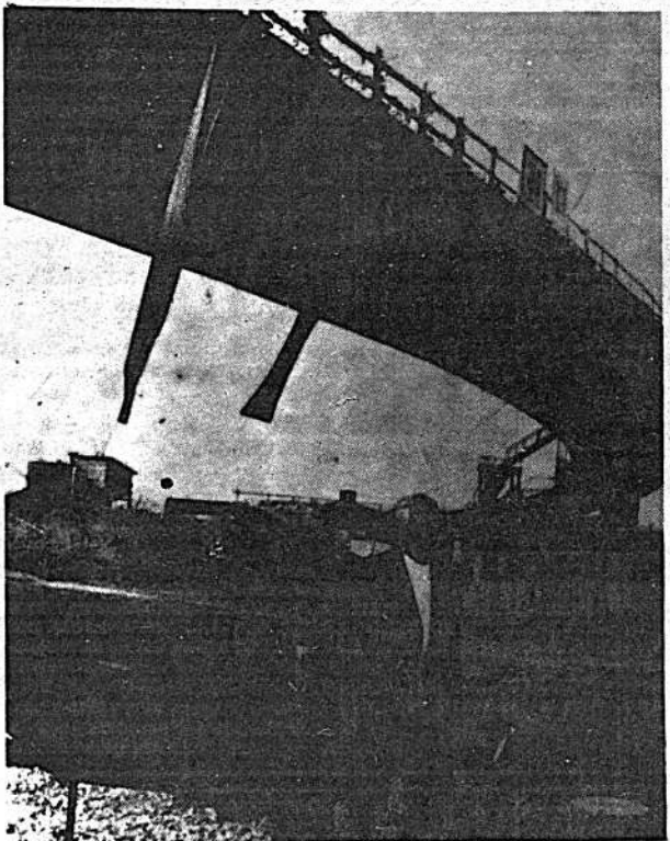
El mayor puente de Europa de "una sola pata", de 470 metros de longitud, será entregado al tránsito, según está previsto, durante el verano de este año. El puente está en el terreno olímpico de "Oberwiesefeld", en Munich, Alemania Federal.
