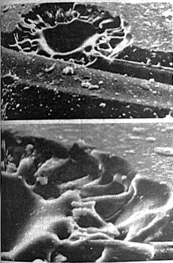
PEQUEÑOS CRATERES. — Estas altamente magnificadas fotos de trozos lunares, muestran un microcráter "zap" aparentemente formado por la alta velocidad de impacto de una partícula de polvo. El cráter de arriba está aumentado en 3.400 veces y el de abajo en 9.700. Las fotos fueron hechas en Pasadena, por los doctores G. J. Wasserburg, J. Devaney y K. Evans, del Laboratorio de Propulsión Jet. (AP Wirephoto).
