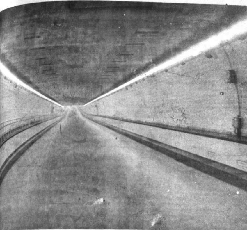
Una vista del Túnel Subfluvial de la Provincia de Santa Fe. El interior del túnel está iluminado por células fotoeléctricas, que permite el acostumbramiento gradual a los conductores.
