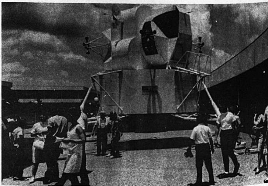
MODULO LUNAR. — Antes del lanzamiento de Apolo 11, en el Centro Espacial de Vuelos Tripulados fue exhibido un vehículo similar al Módulo Lunar que será utilizado para el descenso en la Luna. Numerosas personas admiraron la complejidad del aparato llamado "Araña". (AP Wirephoto).—
