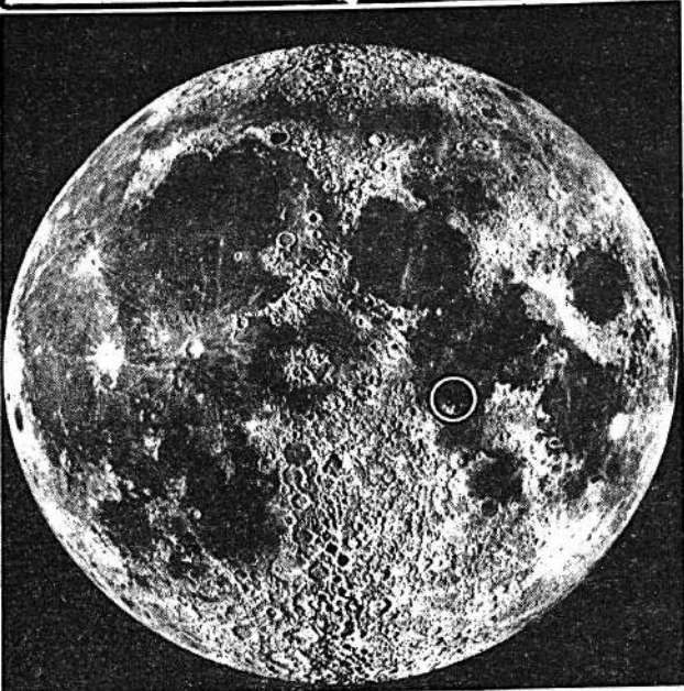
META DE APOLO 11.— Esta es una composición fotográfica de la Luna con un círculo marcando el sitio del proyectado alunizaje de Apolo 11 en el Mar de la Tranquilidad. La fotografía, mostrando la Luna de la primera hasta su última parte, fue lograda por el Observatorio Lick, cerca de San José California. (AP Wirephoto).—
