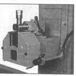
Un diamantador manual fabricado por Ferdimat Industria y Comercio de Máquinas Operadoras Ltda. (FERDIMAT) del Brasil.
