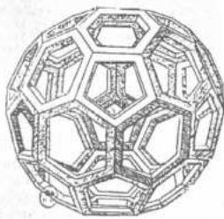
El poliedro semirregular que dibujó Leonardo da Vinci para Fra Luca Paccioli.
