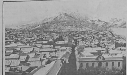
El Cerro de Potosí El legendario y majestuoso "Cerro de Potosí, declarado por UNESCO como "Patrimonio de la Humanidad", es motivo de un estudio técnico e histórico en una mesa redonda que se realiza en Potosí, con participación de expertos geólogos que se debe preservar por sobre todas las cosas" la estructura física de esa cumbre.
