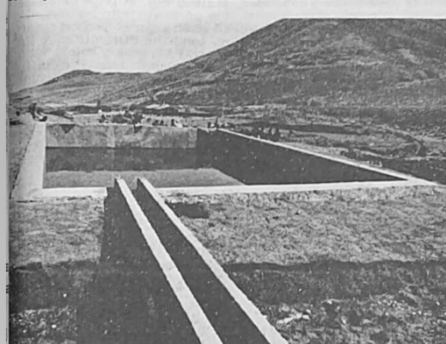
Producción garantizada... Este sistema de microriego garantizará la producción de hortalizas, incluso durante las épocas de sequía...
