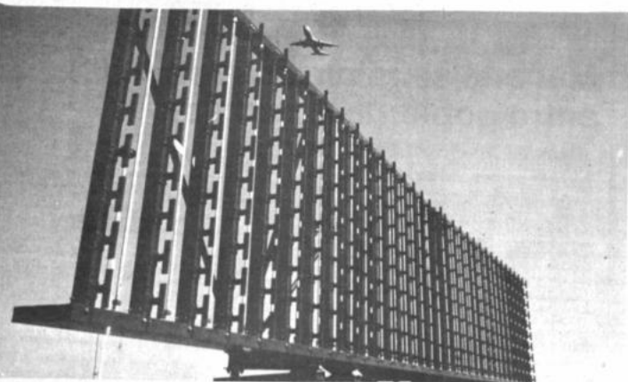
Radar secundario donado por España, que es utilizado en el país para control de la aviación comercial.
