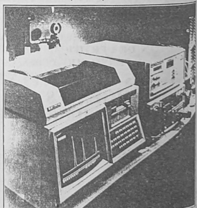
Chromatografía líquida de Alta Presión. Shimadzu Modelo LC-6A Detector ultravioleta visible SPD-6A y Microprocesador Chromatopac CRA4. Perteneciente al Departamento de Biodisponibilidad Farmacéutica de Laboratorios Recalcine Internacional.
