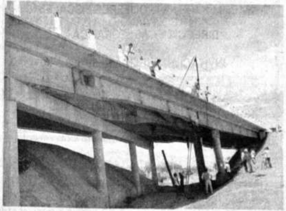
VIADUCTO A COTOCA. SANTA CRUZ, 8 (PRESENCIA). El puente o viaducto de Cotoca que presenta daños en su estructura, la sugerencia para habilitarlo para el uso de vehículos livianos, ha causado polémica. Santa Cruz está exigiendo se determinen responsables de esta obra con fallas que tuvo un sobrepeso de casi el cien por ciento. Otras opiniones, aseguran que resultará más barato al país construir otro puente que reparar el deteriorado. El viaducto tenía poco más de un año de servicio. (Foto PRESENCIA Santa Cruz).
